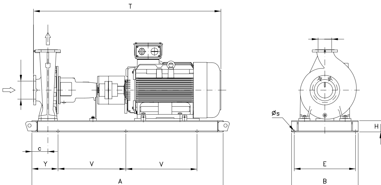
ABB. 2 – GRUNDBLECH – VON 110 kW UND GRÖßER
