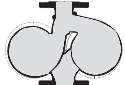
FUNZIONAMENTO IN PARALLELO
