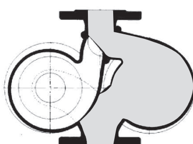
POMPA DESTRA IN FUNZIONE
