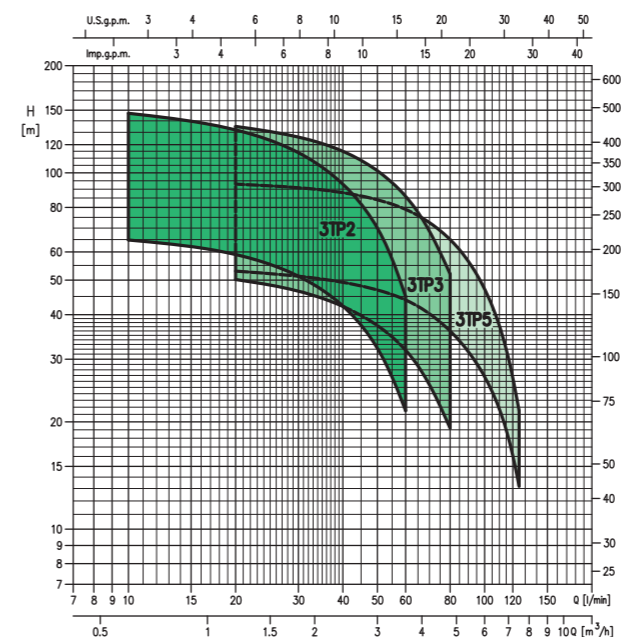
LEISTUNGSKURVE (nach ISO 9906 Anlage A)
